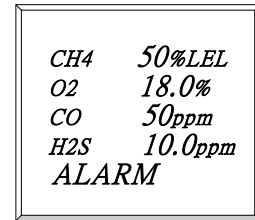
第二警報設定值顯示(ALARM)
