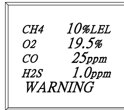
第一警報設定值顯示(WARNING)
