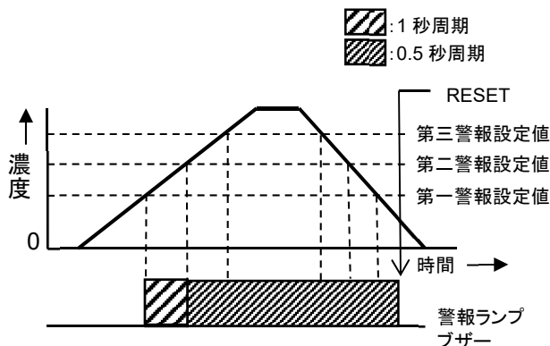
酸素以外の場合 『警報パターン(H-HH-HHH)』
