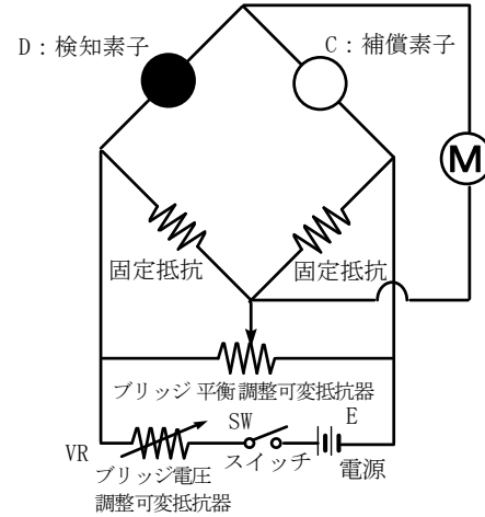
基本回路
