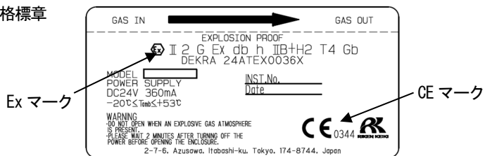
ATEX, CE マーキング仕様の銘板例 (DC 電源仕様のみ)
