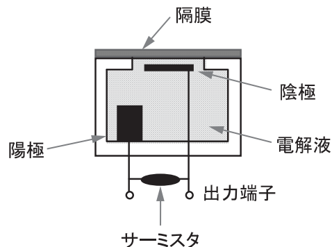
<構造図>
