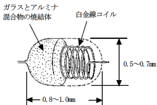
構造図
